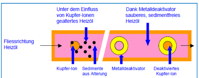
Abbildung 2: Wirkungsweise Metalldeaktivator
